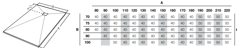
MEDIDAS ESTÁNDAR DISPONIBLES Y DISTANCIA A VÁLVULA STANDARD MEASURES AVAILABLE AND DISTANCE TO VALVE / MESURES STANDARD DISPONIBLES ET DISTANCE À LA VANNE MISURE STANDARD DISPONIBILI E DISTANZA DEL SIFONE / VERFÜGBARE STANDARDGRÖßEN UND ENTFERNUNG ZUM ABLAUF
